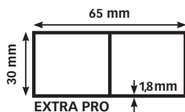
Rechthoekig profiel "bouw" GEANODISEERD Profil rectangulaire pour "maçon" ANODISÉ
