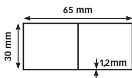
Rechthoekig profiel "bouw" Profil rectangulaire pour "maçon"
