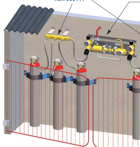
Grille de protection Metal protection grill
