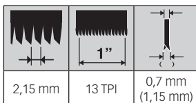
Handzaag MAGNUM 300 • Scie égoïne MAGNUM 300
