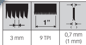
Inklapbare zaag "G-SAW 240" • Scie pliante "G-SAW 240"
