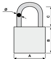
Cylinderhangslot EUROTOP - massief messing - EN-12320 Cadenas à cylindre EUROTOP - laiton massif - EN-12320
