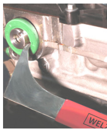
4309-WW Dichtringen-bourrage trekker & plaatser. Outil pour extraire et placer les bourrages Ø 46 - 60mm
