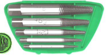
KUKKO49-A 5 St./Pc. M3-M18 38 € KUKKO49-B 6 St./Pc. M3-M24 46 € KUKKO49-C 8 St./Pc. M3-M45 93 €
